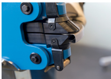
Stauchen von U-Profilen mit geringer Steghöhe / Shrinking low webbed U-profiles
